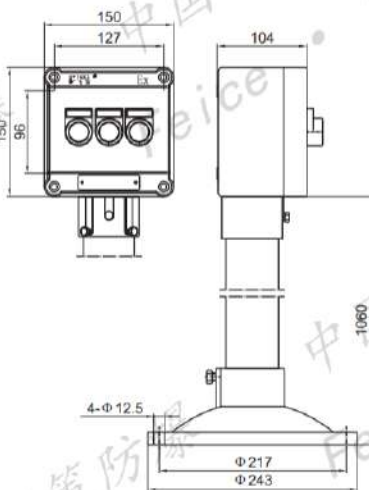
1型(立式) Type 1 (vertical)
