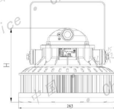
SFCG71-g-III型 (支架式Z)
