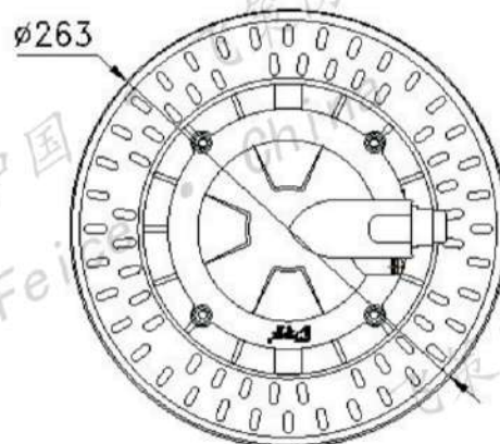
SFCG71-III型 (平台式P)
