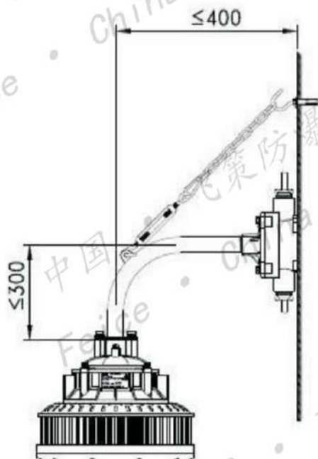
壁式90° (B2) / 配接线盒
