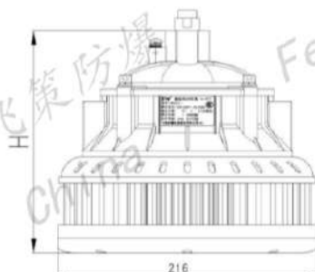
SFCG71-g-II型 SFCG71-g-II Type
