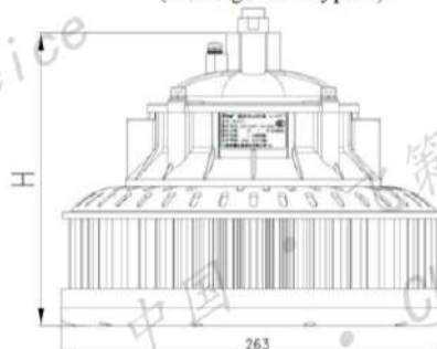
SFCG71-g-III型 SFCG71-g-III Type
