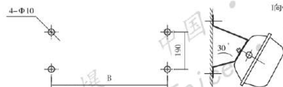
(B1) 壁式 Wall type
