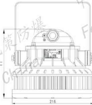
SFCG71-g-II型 (支架式Z)
