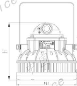
SFCG71-g-I型 (支架式Z)
