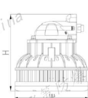
SFCG71-g-I型 (平台式P)
