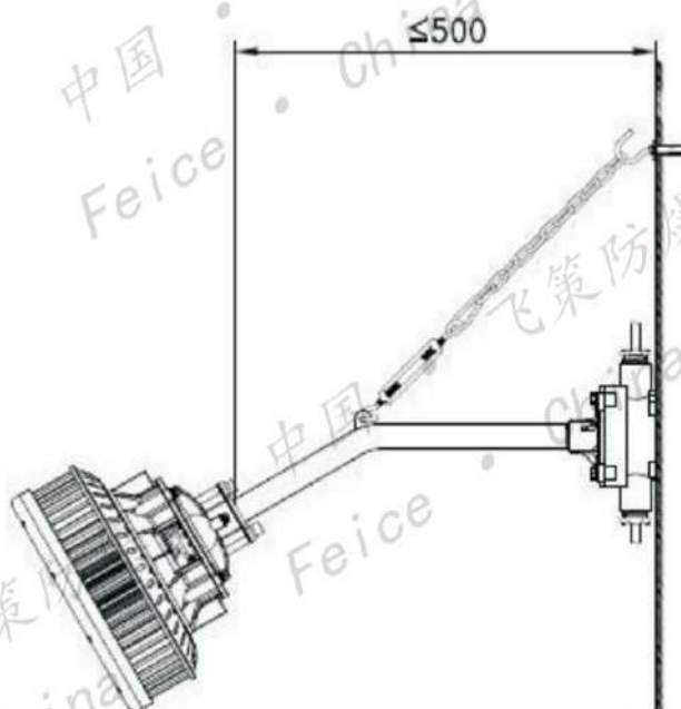
壁式30° (B1) / 配接线盒
