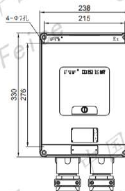
40A、50A、63A小型断路器(3P/4P) 40A, 50A, 63A miniature circuit breaker (3P/4P)
