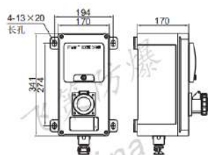
1型16A插销 1Type 16A latch
