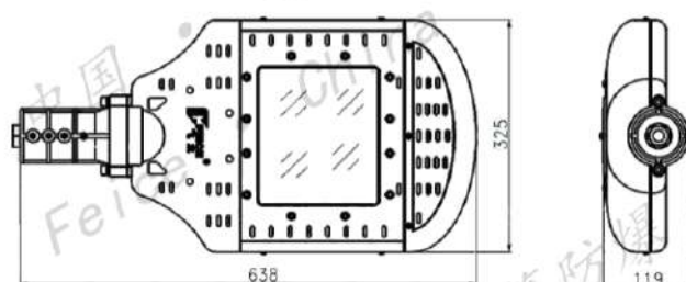
2.路灯式 Street lamp type
