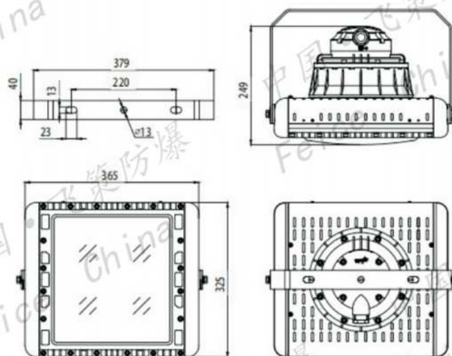
FCF(T, L) 98-(200W-240W)
