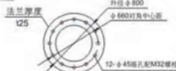
法兰平面示意图 Flange plane schemes
