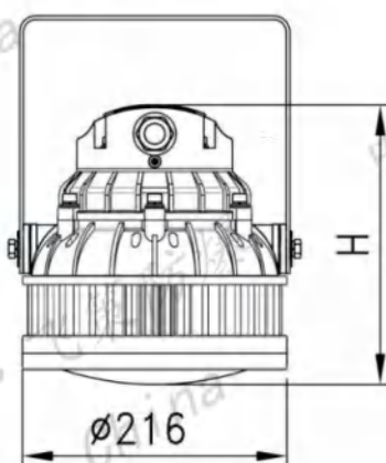
II型支架式 Type II stents type
