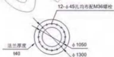
法兰平面示意图 Flange plane schemes
