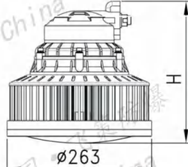
III型平台护栏式 Type III platform guardrail type
