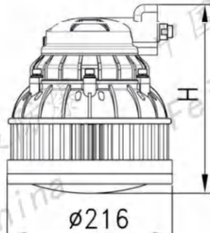
II型平台护栏式 Type II platform guardrail type
