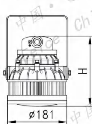
I型支架式 Type I stents type
