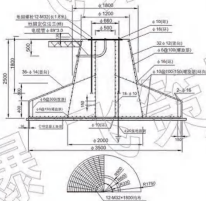
15~20m高杆灯 High-pole lamp 基础平面图 Foundation plan
