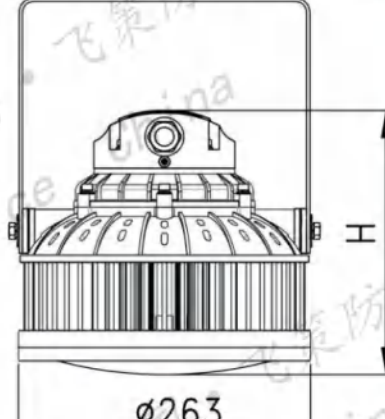
III型支架式 Type III stents type
