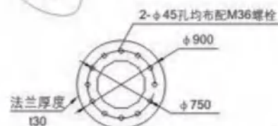
法兰平面示意图 Flange plane schemes
